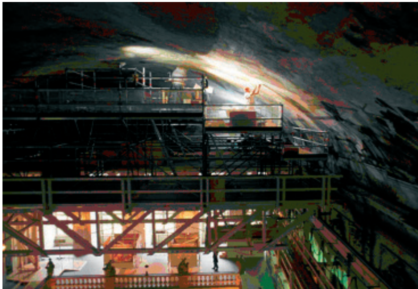
Abb. 1: Das Brückengerüst wurde bereits 1995 konstruiert und zur Notfestigung des Freskos sowie zur Untersuchung der Maltechnik verwendet. Es ist auf Schienen gelagert und kann mittels Synchronantrieb bewegt werden. Ein weiteres Brückengerüst und ein Standgerüst schaffen ab 2003/04 ausreichend Arbeitsplätze für die Restauratoren, ohne das gesamte Tiepologemälde einrüsten und damit verdecken zu müssen.
